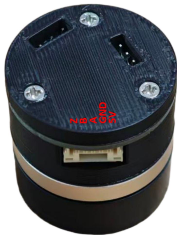
增量式编 码器接口
