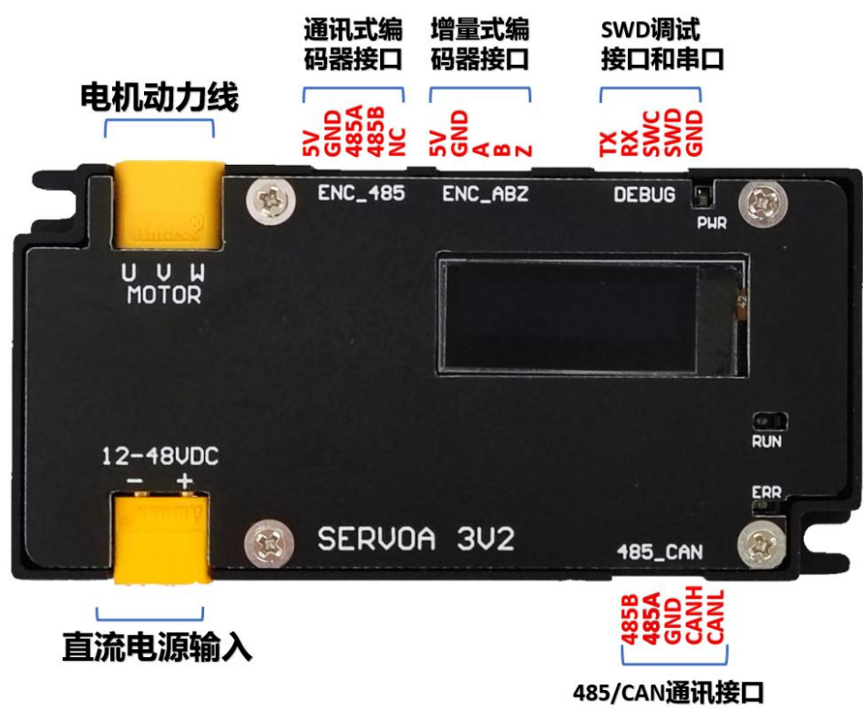
驱动器接口图
