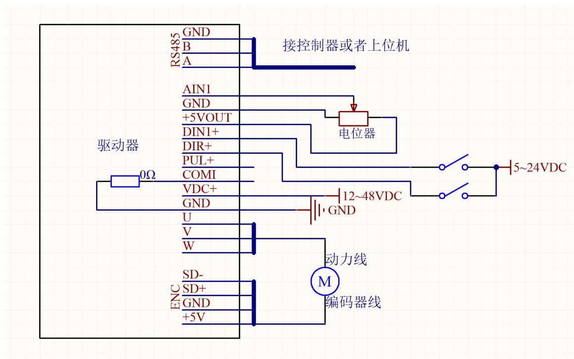
接线图
